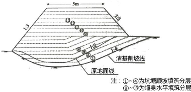
图 4 围堰横断面分层填筑示意图
